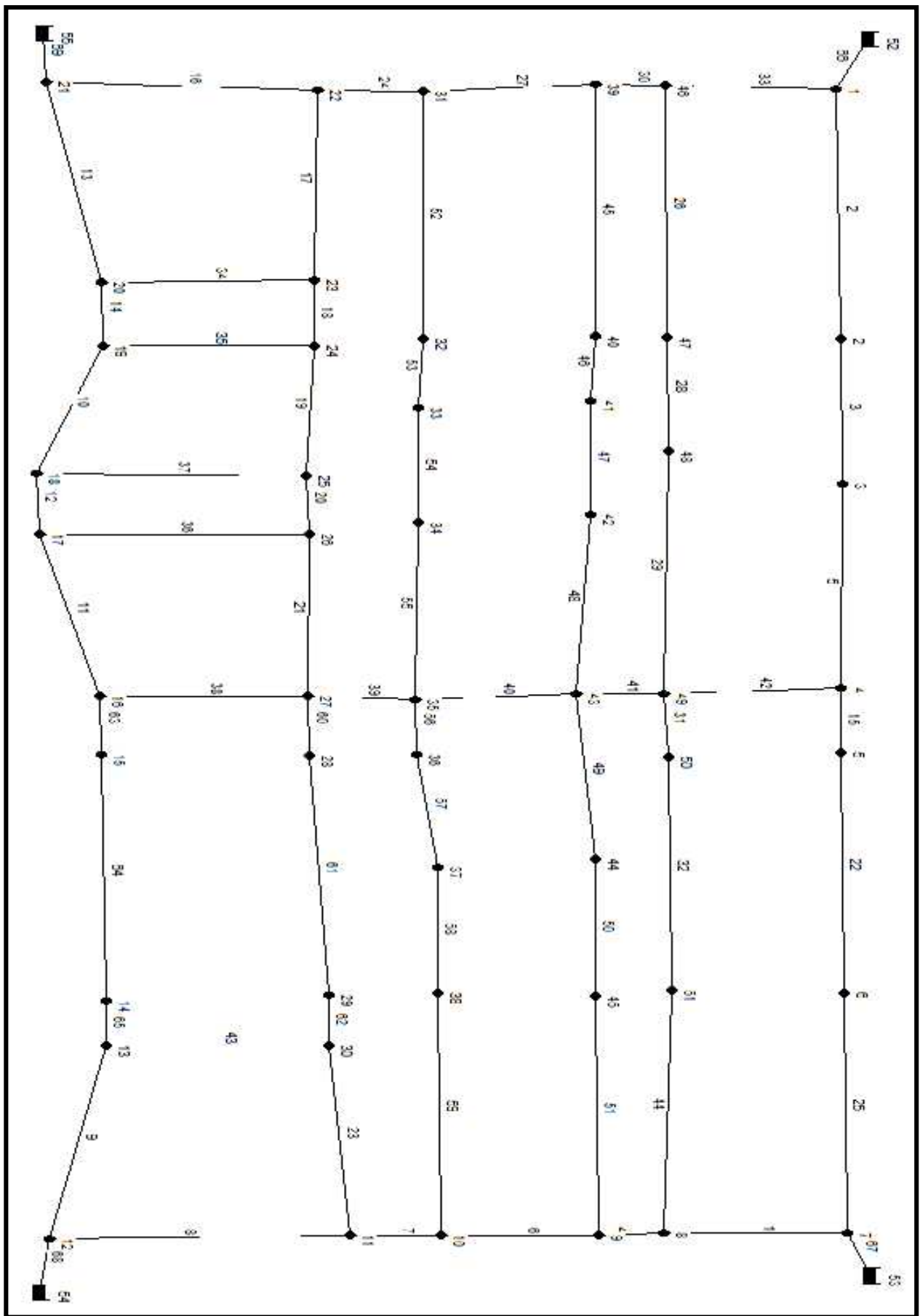
Figure II.12: Réseau de distribution d'eau potable du lotissement.
