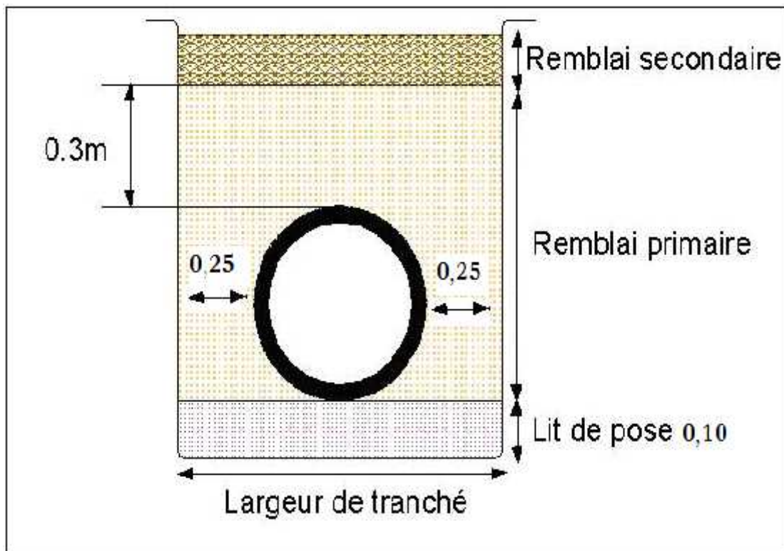
Figure II.11: Coupe type de la tranchée.
