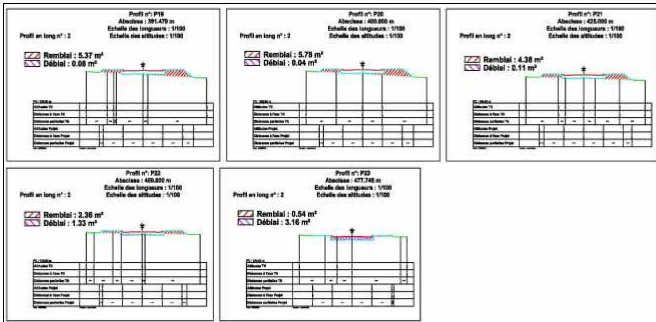
Figure II. 8: Profils en travers du profil en long de la voie n°2.
