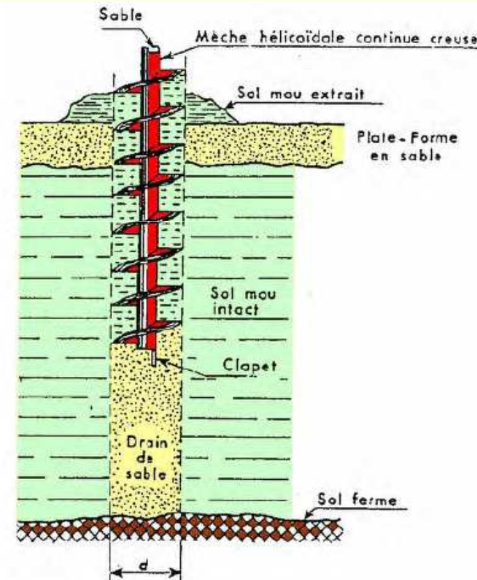
a - Réalisation d'un drain de sable par forage à la tarière à âme creuse
