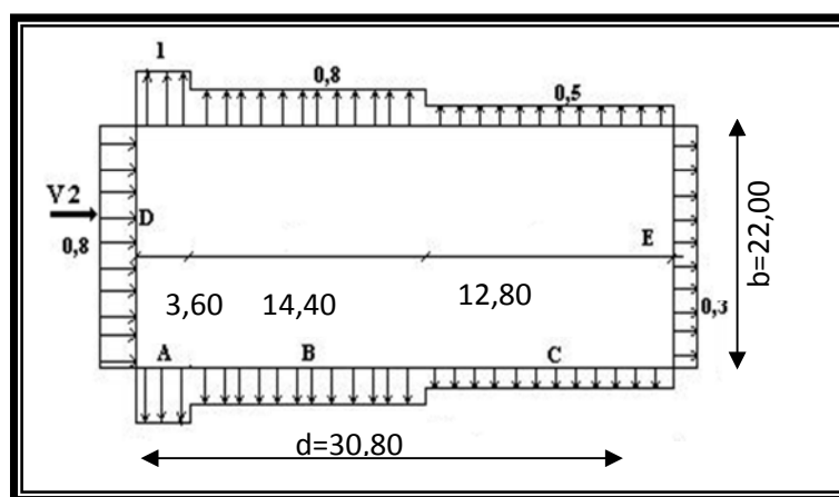
Figure III.9 : Valeurs de Cpesurlesparoisverticales.DirectionduventV2
