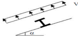
Figure V.4 : Cas de l'effet du vent
