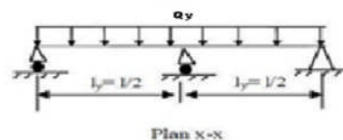
Figure V.6 : Cas de la charge max Q_y ; Q_z
