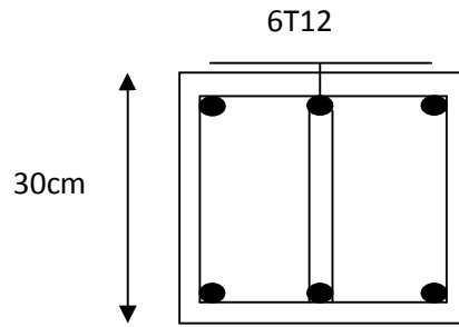
Figure. X.6 : Ferrailage de la longrine
