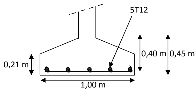
Figure. X.5 Ferrailage de la semelle d'angle
