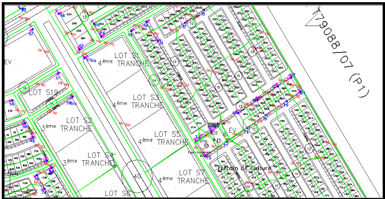
Figure 24 : Exemple du tracé des zones nodales
