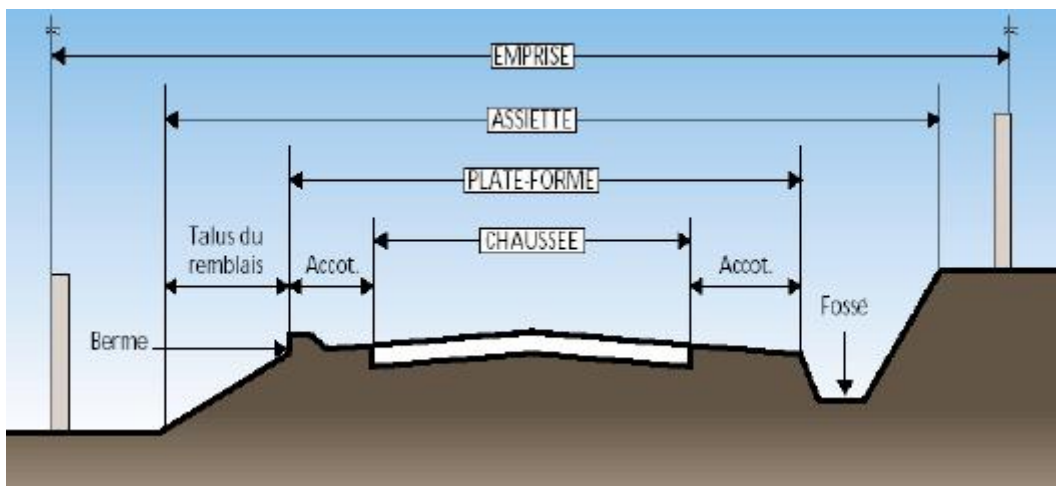
Figure 3: coupe horizontale d'une voie
