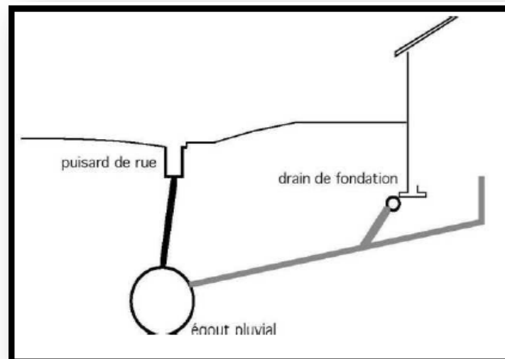
Figure 11:présentation schématique des branchements (En Système unitaire)
