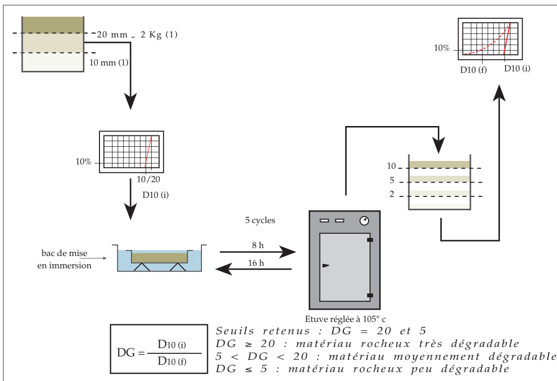
Figure 2 : Principe de l'essai de Dégradabilité (DG)
