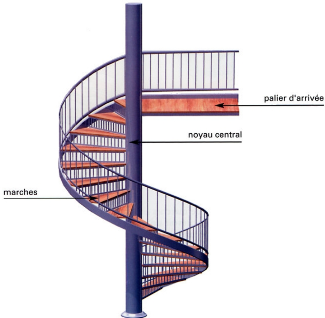
Figure 6.8 : Escalier hélicoïdal
