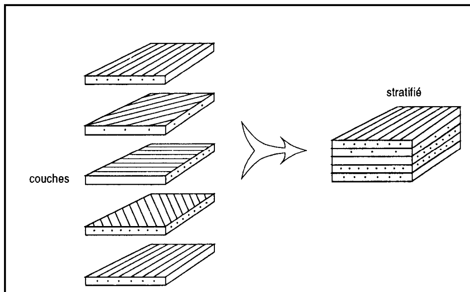
Fig. (I.9) : Constitution d'un stratifié
