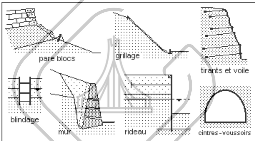
Figure 4.3.2.1.6 – Ouvrages de soutènement
