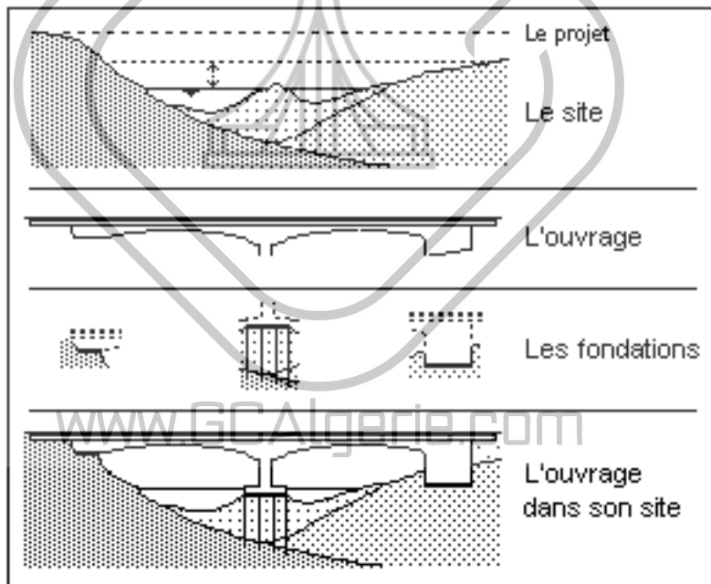
Figure 2.4.2 – Le projet, le site et l'ouvrage
