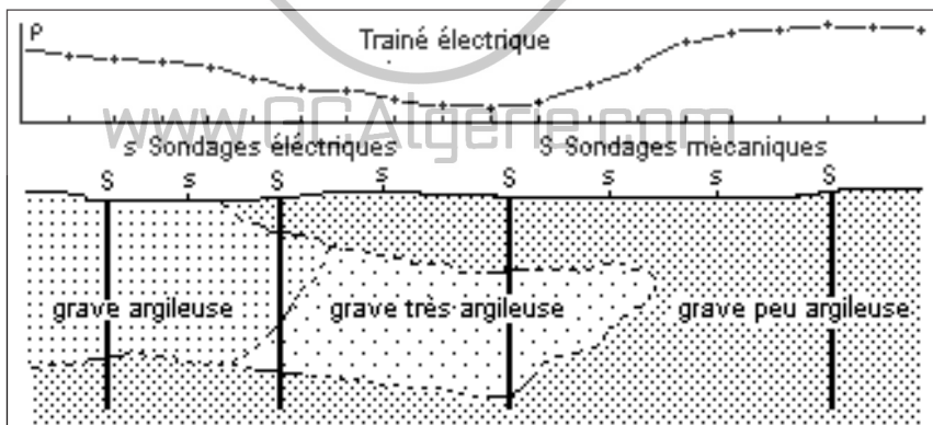
Figure 1.4 – Hétérogénéité d'une grave plus ou moins argileuse
