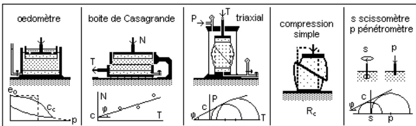
Figure 5.5.4.2 – Essais mécaniques de laboratoire
