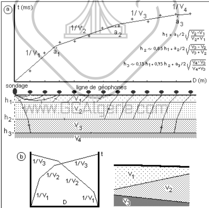
Figure 5.5.2.3.1 – Sondages de sismique réfraction
