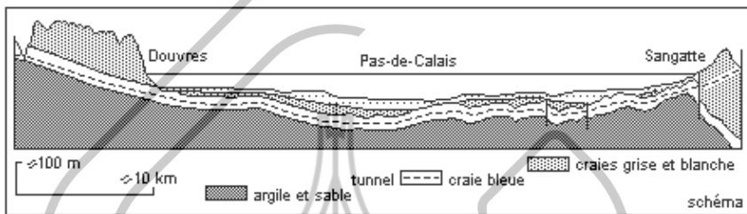
Figure 4.5.1.3 – Le tunnel sous la Manche
