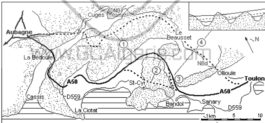
Figure 5.3.2.2 – Étude du tracé de l'autoroute A50
