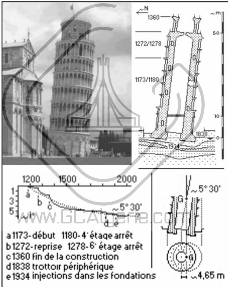
Photo 1.1.2.1 – La tour de Pise
