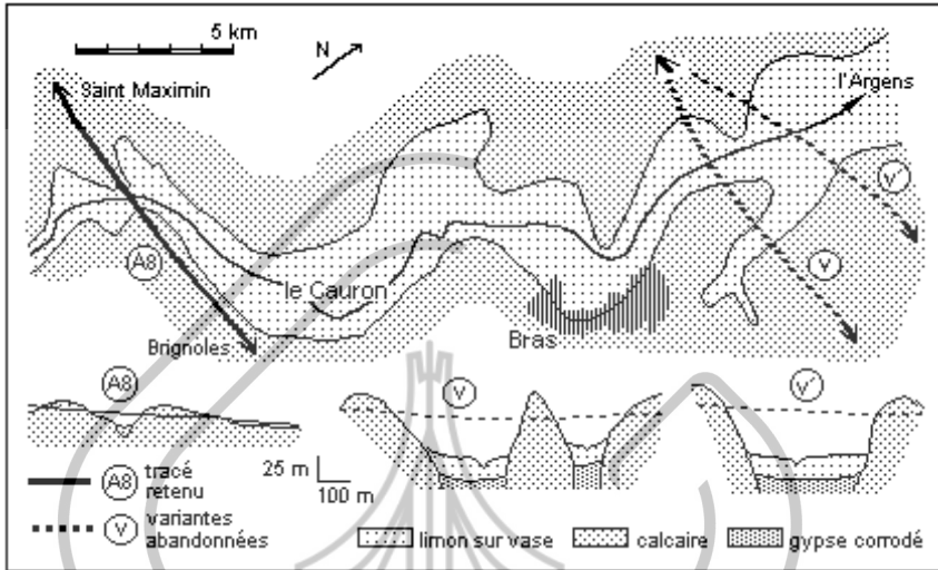
Figure 5.1.1.3 – Autoroute A8 – études de variantes – choix du tracé
