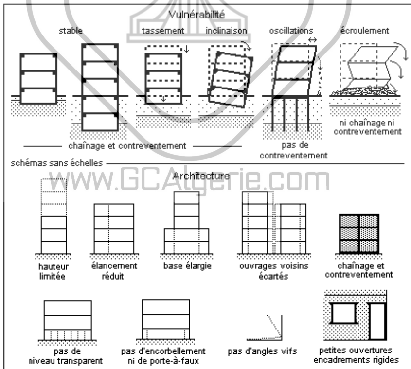
Figure 4.4.3.1 – Génie parasismique
