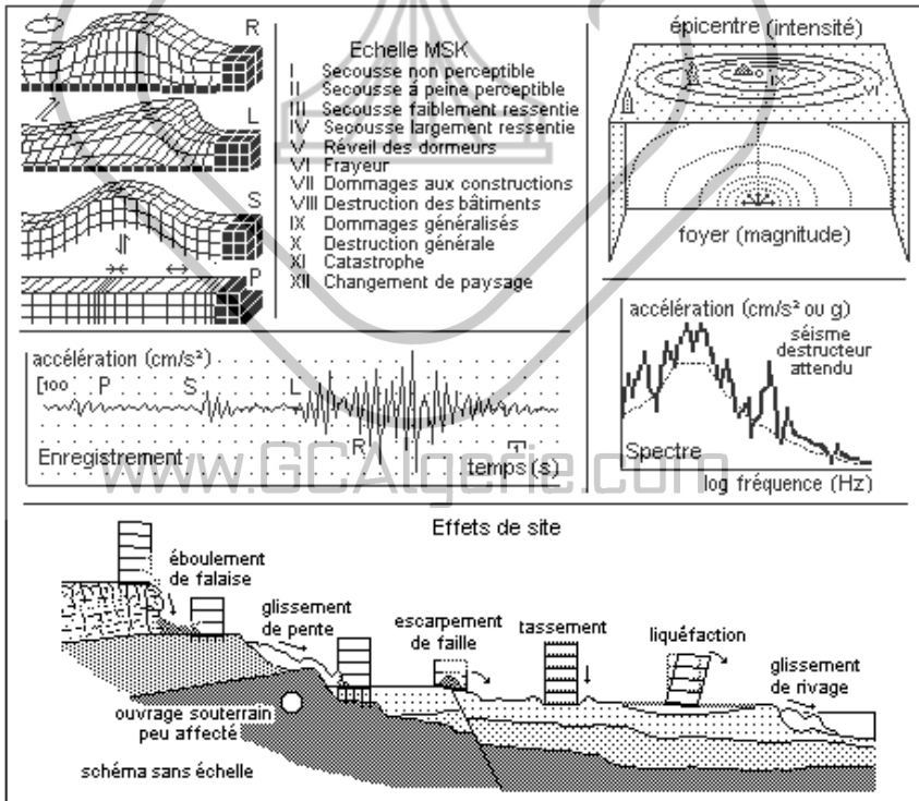
Figure 4.2 - Séismes
