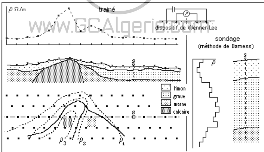
Figure 5.5.2.1 - Résistivité électrique
