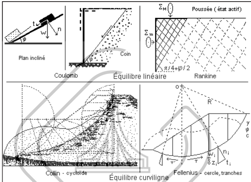
Figure 1.3.4.2 – Équilibres plastiques
