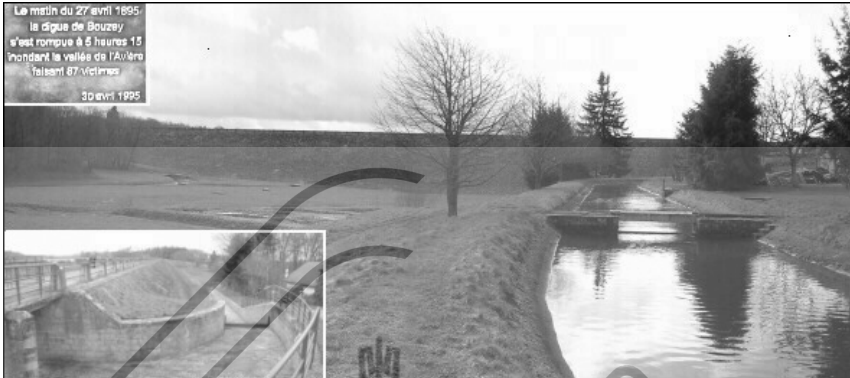
Photo 1.1.1.2 – Le barrage de Bouzey
