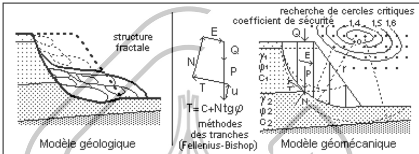
Figure 2.3.2.3 – Stabilité d'un talus
