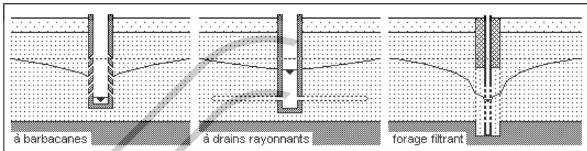
Figure 4.3.2.5 – Types d'ouvrages de captage de nappe
