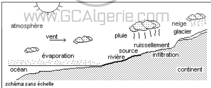
Figure 4.1.2.4 – Le cycle de l'eau
