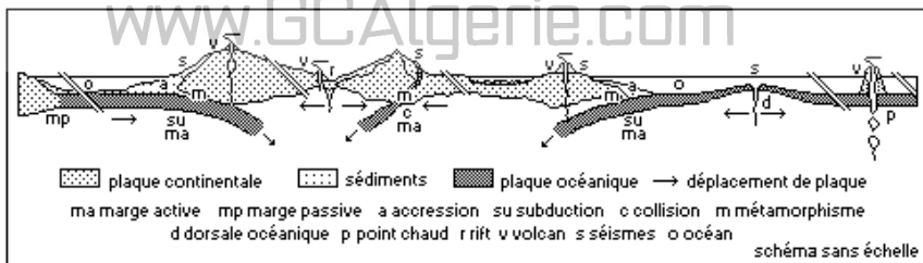
Figure 4.1.2.2.1 – Géodynamique interne
