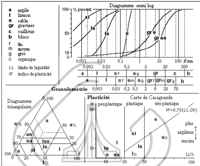
Figure 2.3.1.2- Granulométrie – Plasticité
