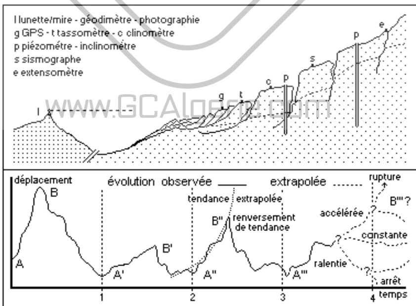
Figure 3.1.2.6 – Évolution d'un glissement de talus
