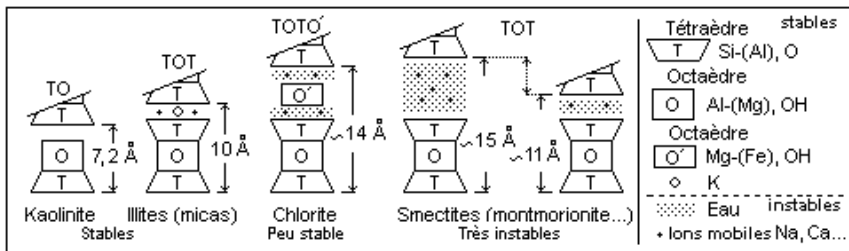
Figure 2.1.2.2.1 – Structures cristallines de minéraux argileux
