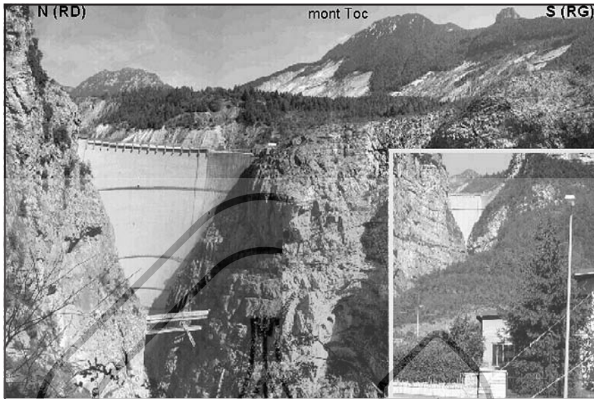
Photo 1.1.1.3.c – Le barrage du Vajont vu de l’aval
