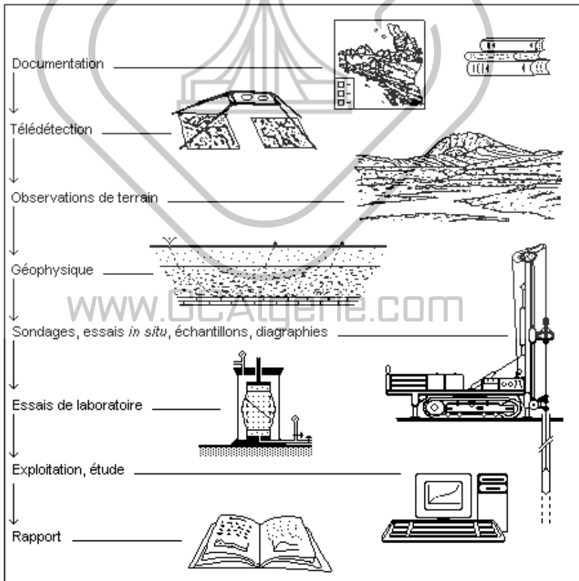
Figure 5.2.3 – Enchaînement des techniques d'étude
