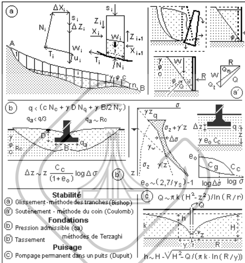
Figure 2.1.1.2.3 – Principaux problèmes de géomécanique
