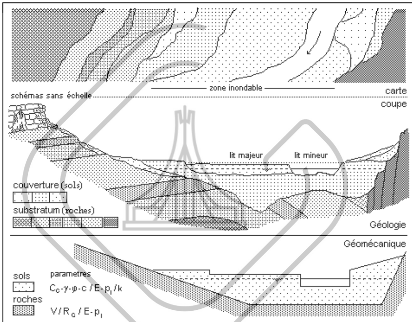
Figure 4.5.2.1 - Modèles de formes
