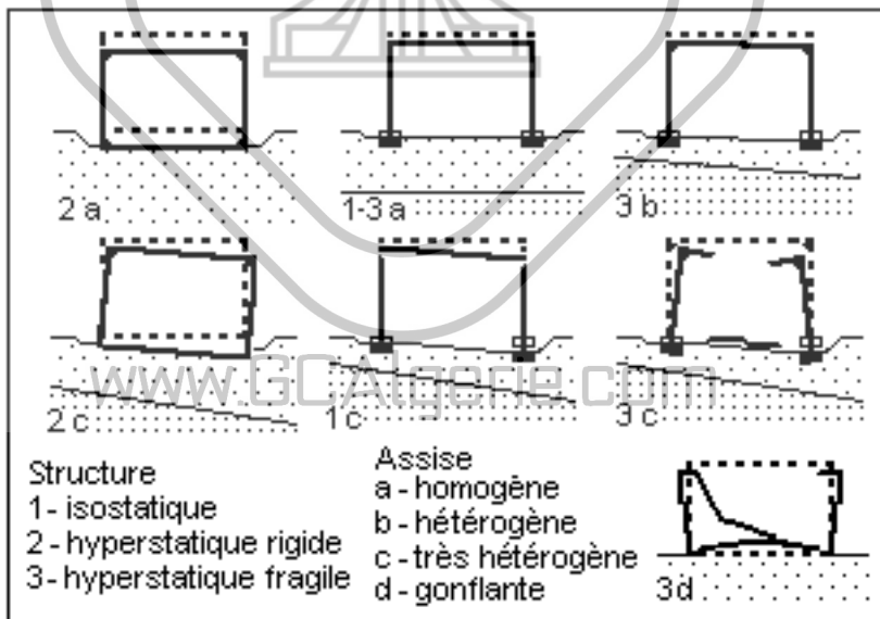
Figure 4.3.2.4.2 – Comportements d'ouvrages mal fondés superficiellement
