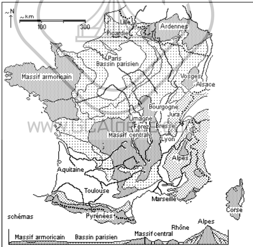
Figure 4.1.3 – Croquis géologique de la France
