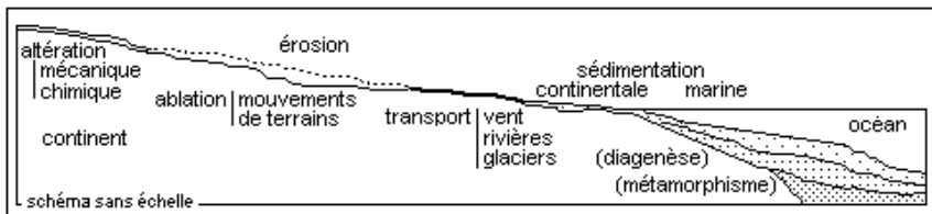
Figure 4.1.2.2.2 – Géodynamique externe
