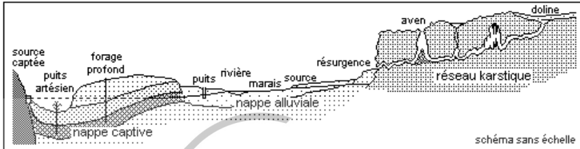
Figure 4.2.6 – Circulations d'eau souterraine
