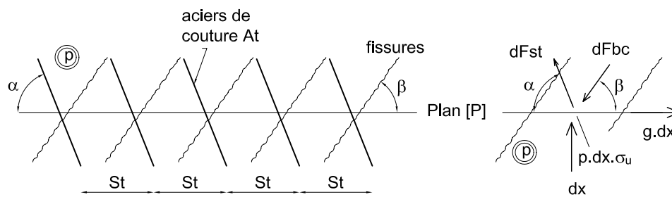
Fig. 41: Equilibre d'une surface élémentaire du plan [P] .
