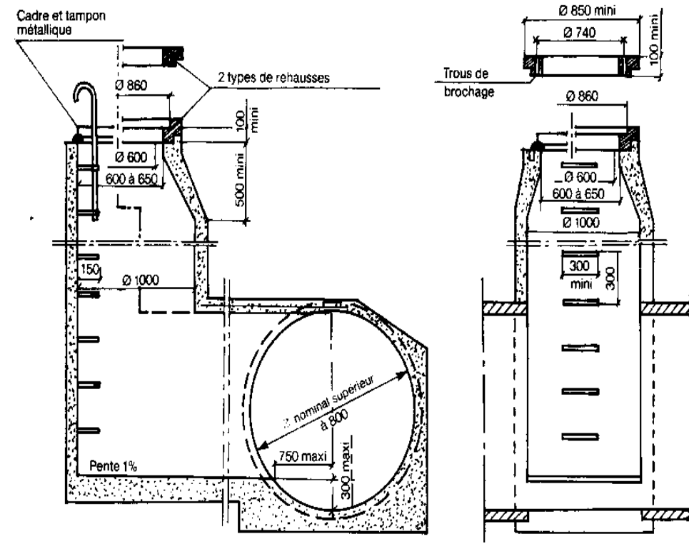
Fig. 57 - Regard de visite à section circulaire de 1 m de diamètre, à accès latéral en dérivation d'une canalisation de diamètre nominal supérieur à 0,80 m. Variantes: avec échelle encastrée, avec échelons saillants.
