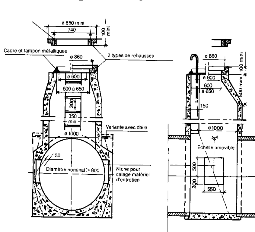
Fig. 56 - Regard de visite à section circulaire de 1 m de diamètre, sur tuyau de diamètre nominal supérieur à 0,80 m. Variantes: avec échelle encastrée, avec échelons saillants.
