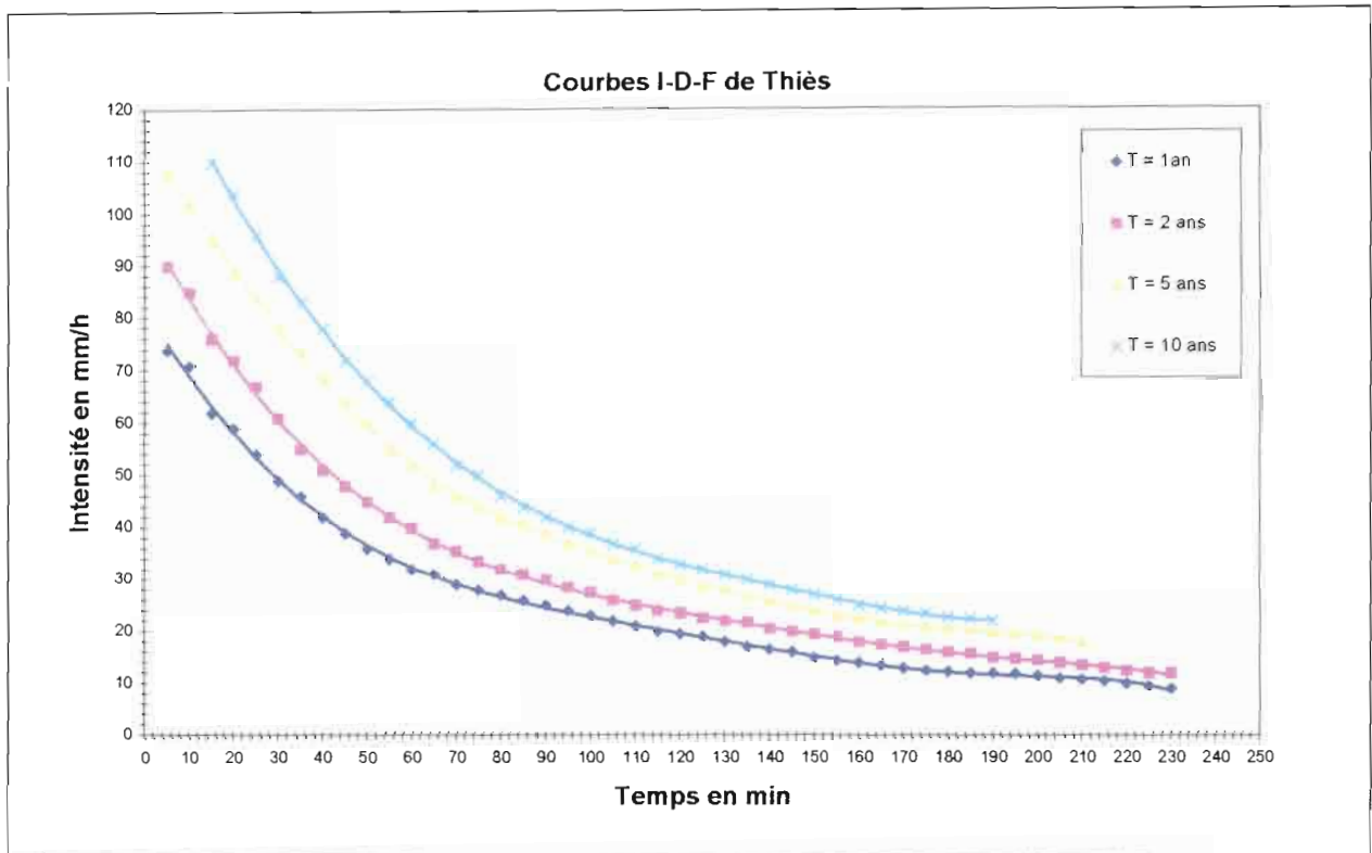
Figure 12 : Courbes I-D-F expérimentales de Thiès (source : ESP_Thiès, Dr Elh. Bamba Diaw)
