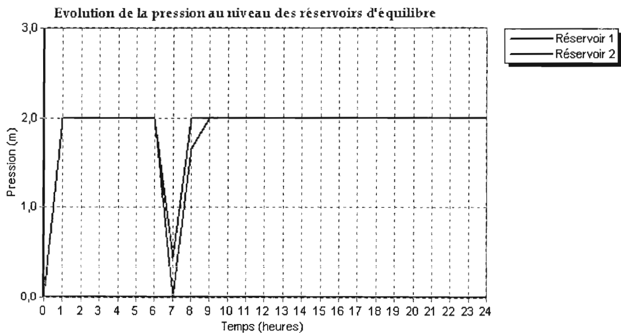
Figure 4 : Evolution du niveau d'eau aux réservoirs d'équilibre.
